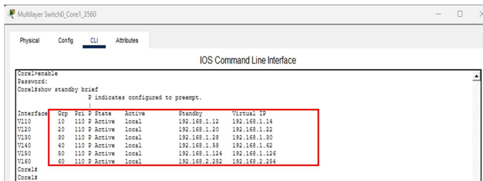
M2-8. ábra – HSRP állapot ellenőrzése Forrás: Saját készítésű képernyőkép
