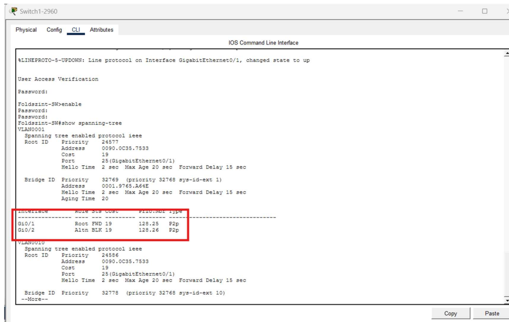
M3-3. ábra – Spanning Tree működésének ellenőrzése Forrás: Saját készítésű képernyőkép
