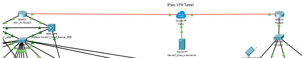
8. ábra Site to site VPN összeköttetés. Forrás: Saját készítésű képernyőkép
